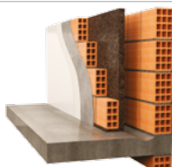
DOBBELT VÆG MED DELVIS UDFYLDNING AF HULRUM
