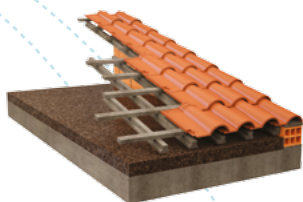
SKRÅTAG MED STIV ISOLERING OVER PLADE
