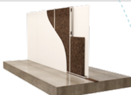
METALSTOLPEVÆG VED AFBRUDT GULVPLADE
