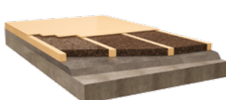
GULVBELÆGNING MED HULRUMSFYLDNING MELLEM GULVBJÆLKER
