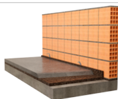
AFKOBLING AF AFRETTERTLAG MOD VÆG
